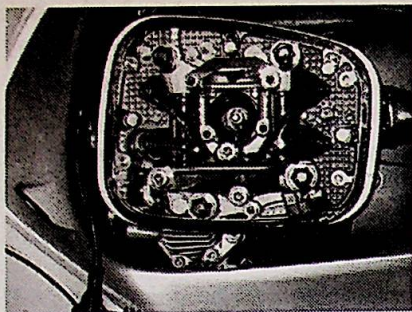
Ventiler på en boxer
